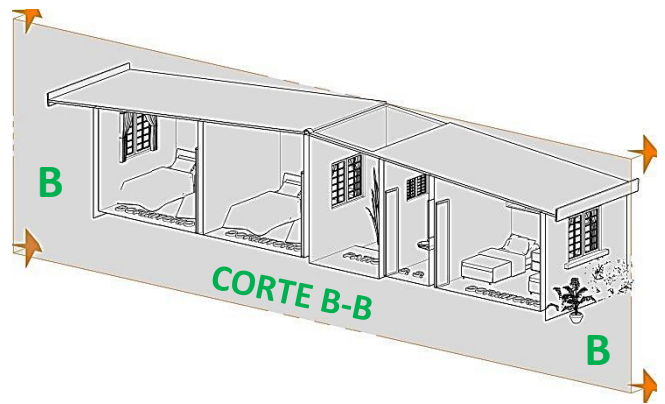
CORTE B-B
