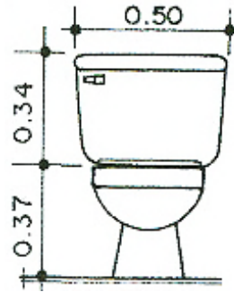
ELEVACIÓN
