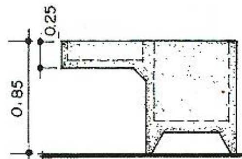
ELEVACIÓN
